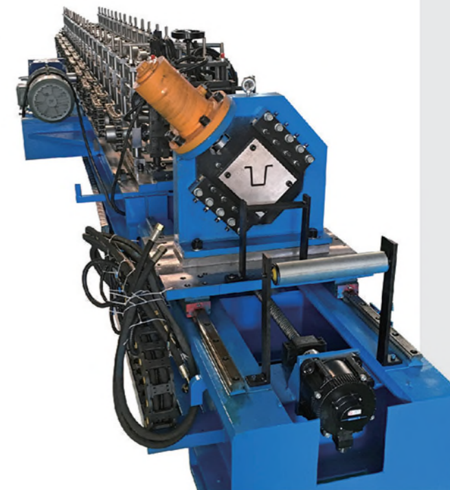
美国通用皮卡底盘加强筋 冷弯成型生产线
